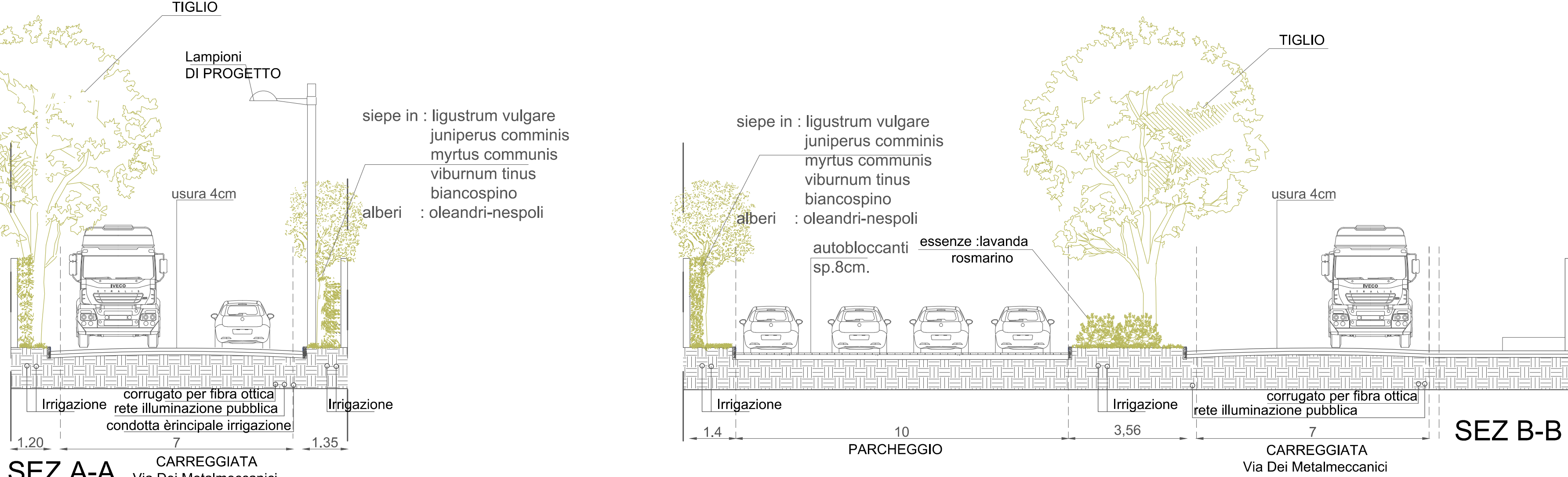
SEZIONI SCALA 1:100
