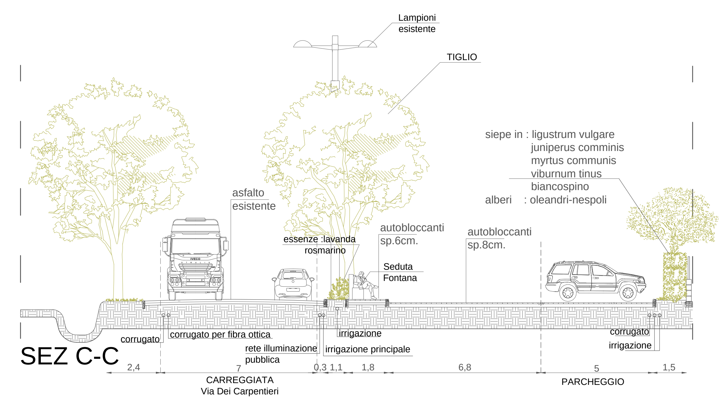
SEZIONI SCALA 1:100
