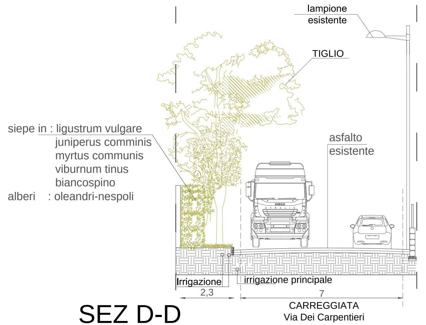
SEZ D-D
